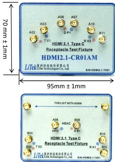
圖 3: HDMI2.1-CR01AM 尺寸圖
